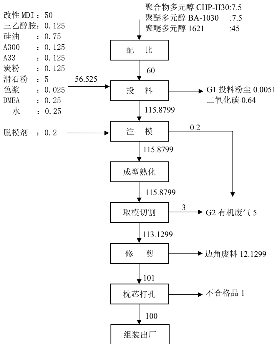
图 3 项目物料平衡图
