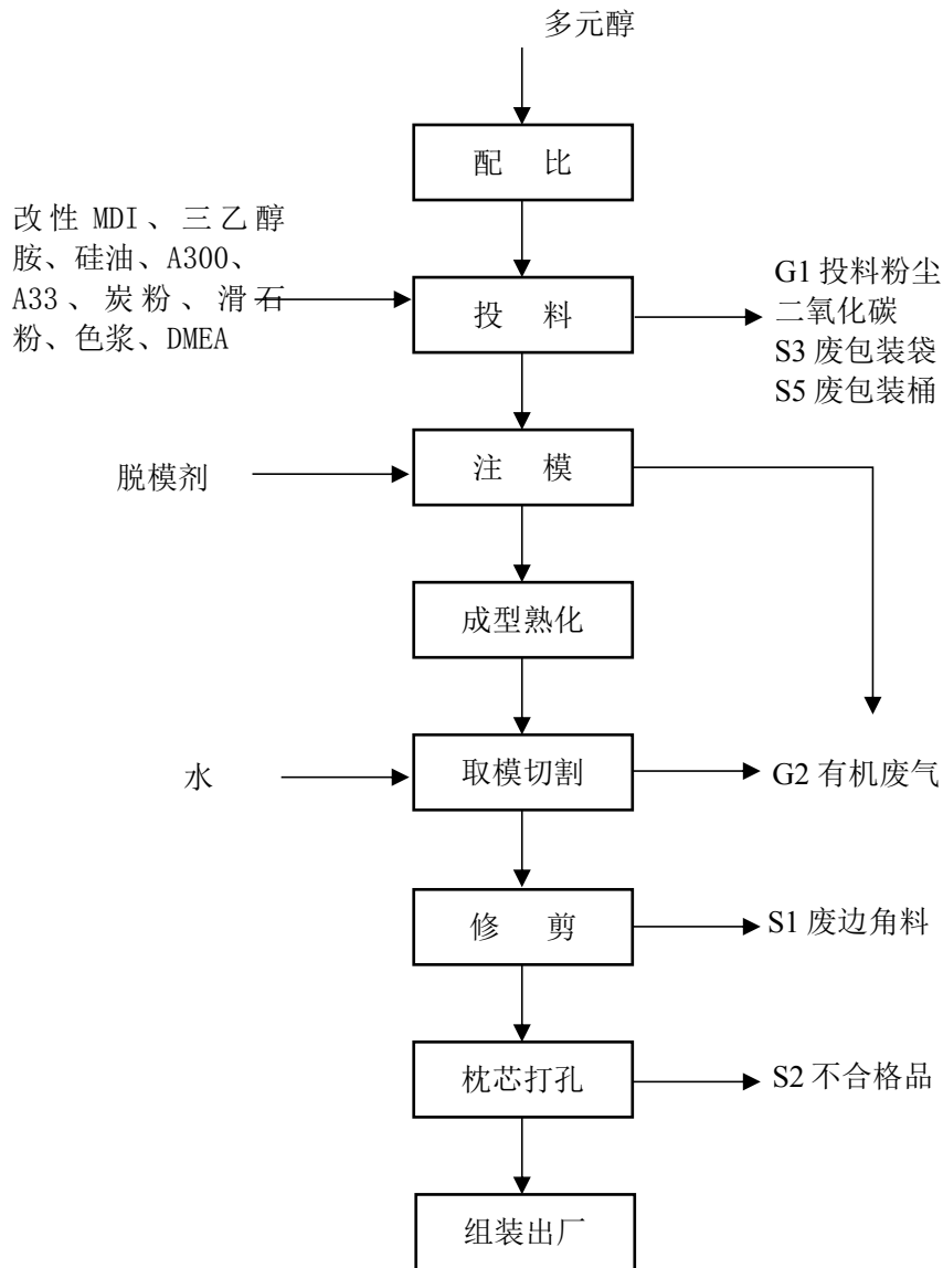
图 2 生产工艺流程及产污节点图
